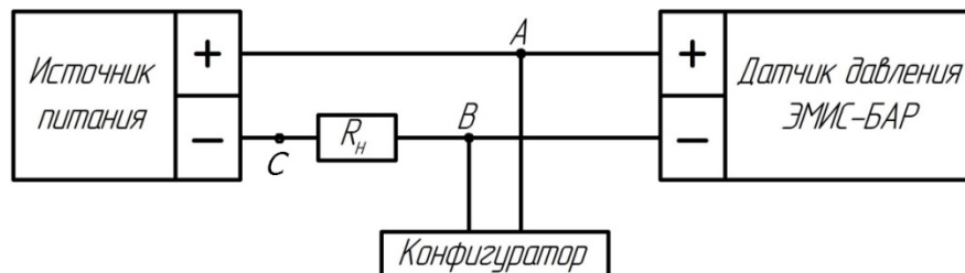
Рисунок 41 – Схема подключения датчика с устройством HART– коммуникации
