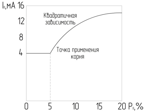
Рисунок 35 – График «КВОБР»
