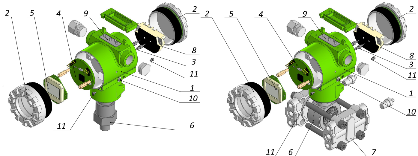
Рисунок 2 – Устройство датчиков давления
