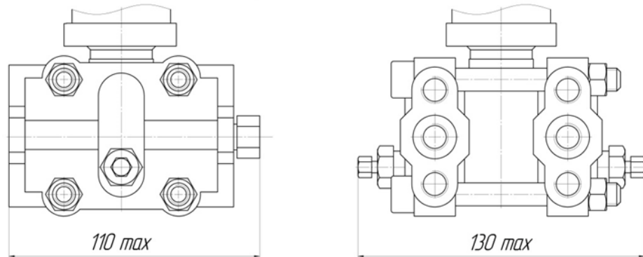
Рисунок Д.3 – Габаритные и присоединительные размеры фланцевого исполнения датчиков давления ЭМИС-БАР 143, 153, 193,105(с диапазонами Hs)
