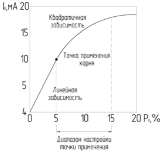
Рисунок 33 – График «КВЛИН»
