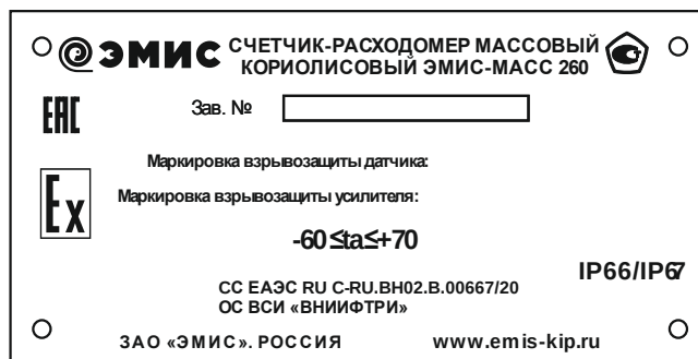
Рисунок 1.4 - Табличка с маркировкой датчика
