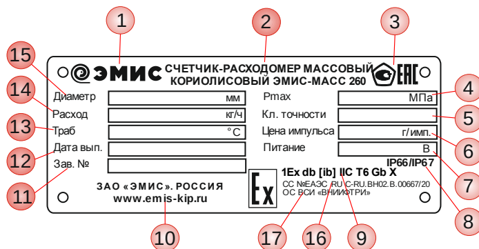
Рисунок 1.3 - Основная табличка расходомера
