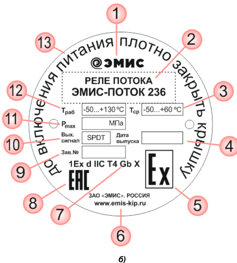
Рисунок 1.4 - Табличка реле потока: а – исполнение без взрывозащиты; б – исполнение с взрывозащитой.
