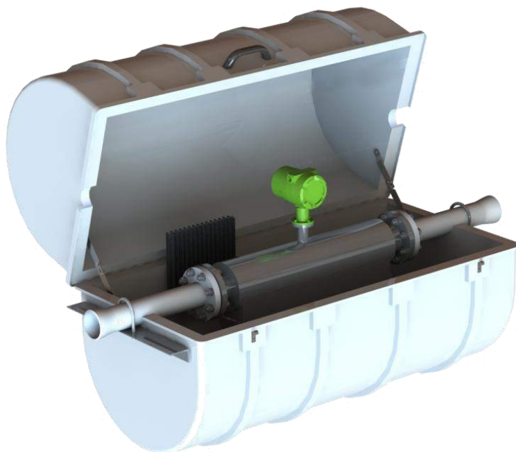
Рисунок 1.3 - Шкаф трубный обогреваемый капсульного типа
