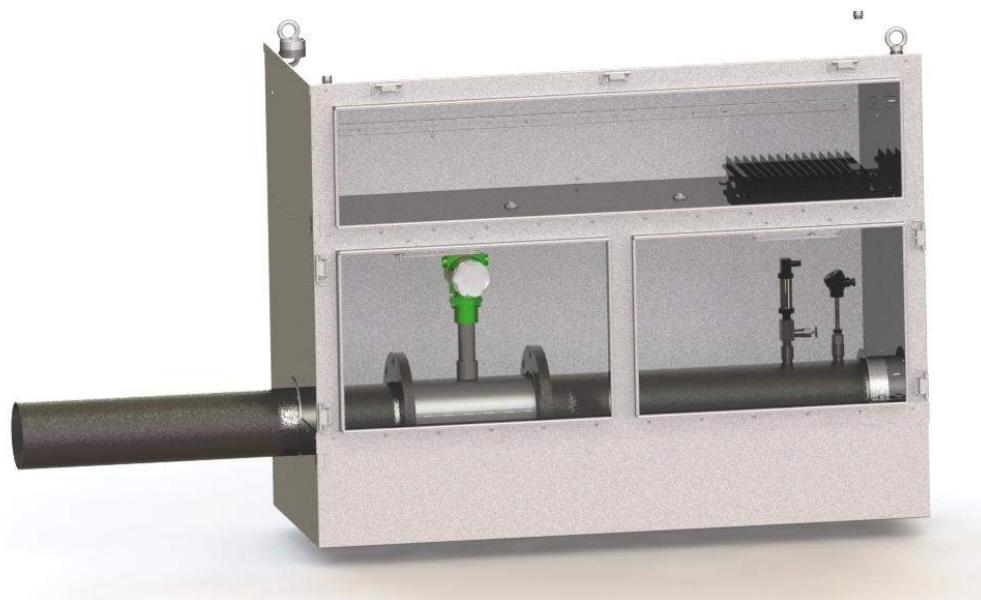
Рисунок 1.2 - Шкаф трубный обогреваемый вертикального типа
