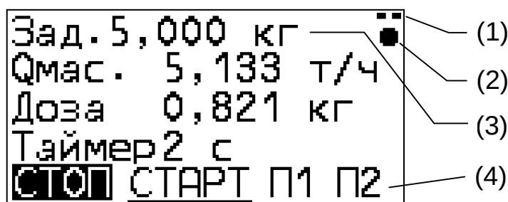
Рисунок 6.11. Панель дозатора.
