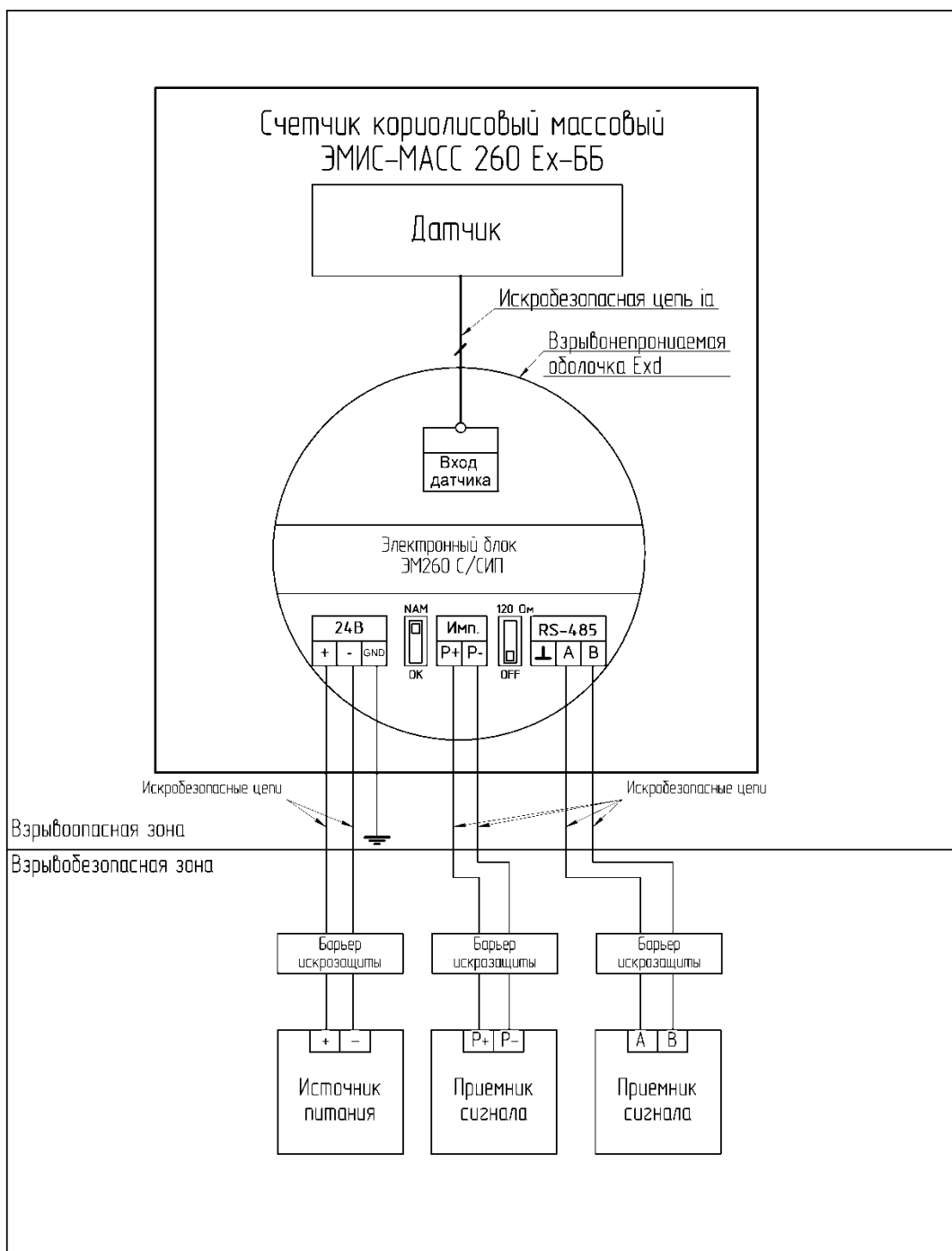
Рисунок 5.3. Электрическое подключение электронного блока исполнения Ex-ББ
