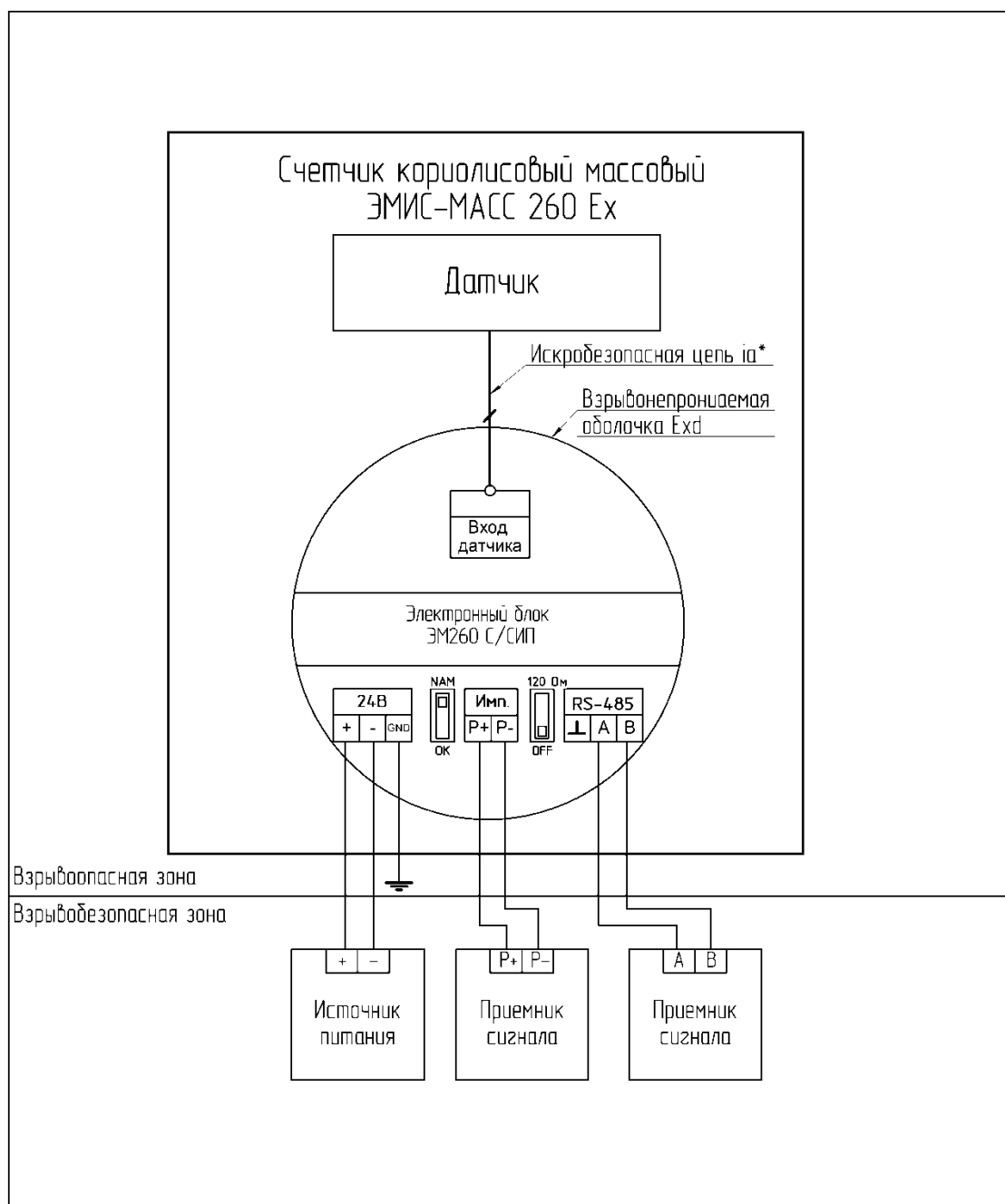
Рисунок 5.2. Электрическое подключение электронного блока исполнения Ех
